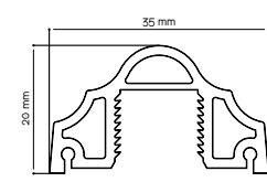
Petite Moulure 35 mm (sans possibilité de vitrer)
