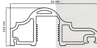
Grande Moulure 54 mm (avec ou sans vitrage)
